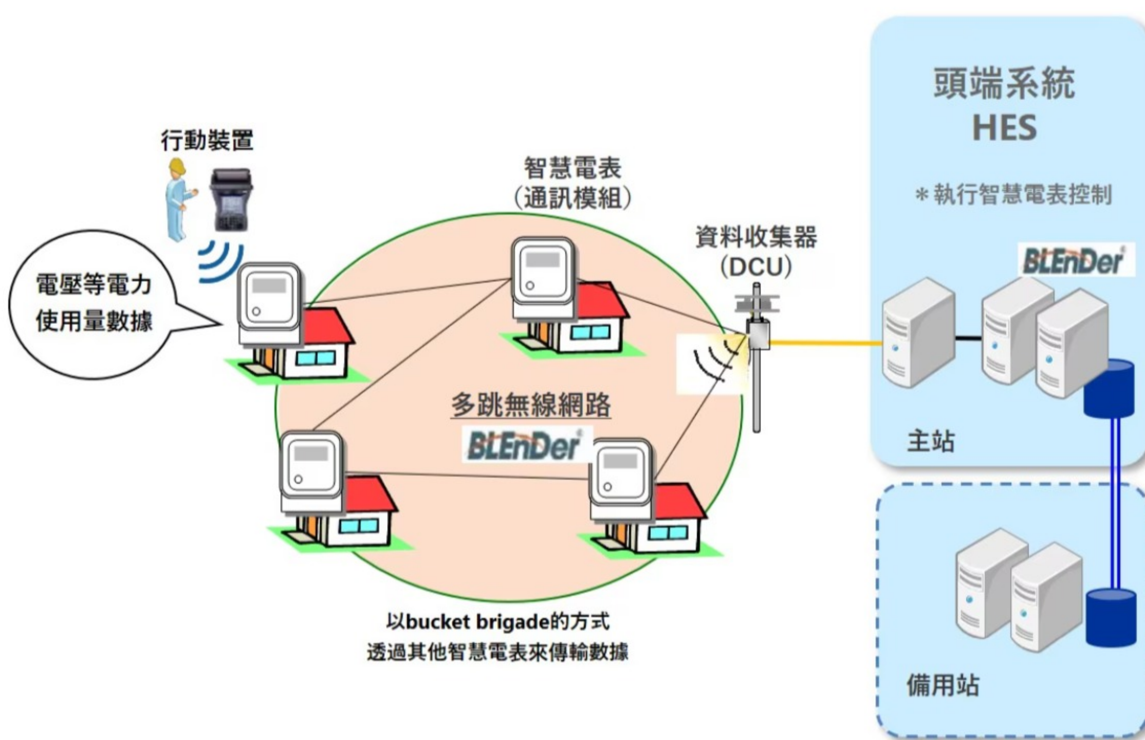
本次智慧電表系統之通訊系統示意圖
